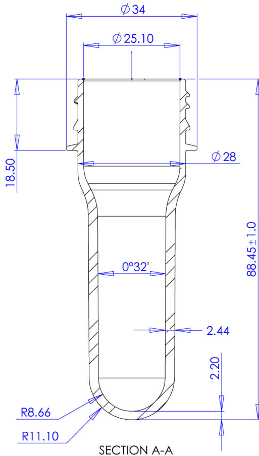
SECTION A-A
