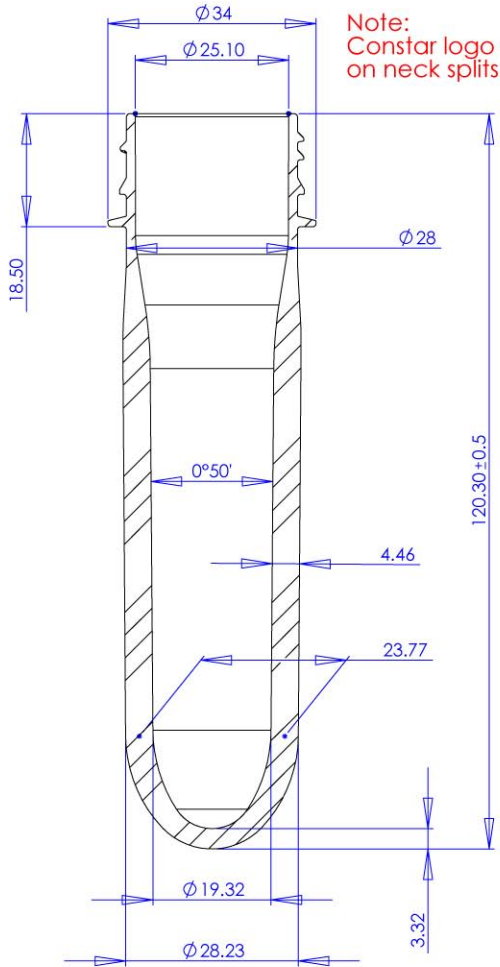
SECTION A-A
