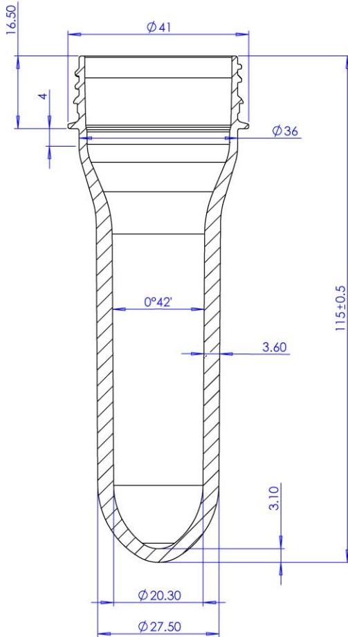
SECTION A-A
