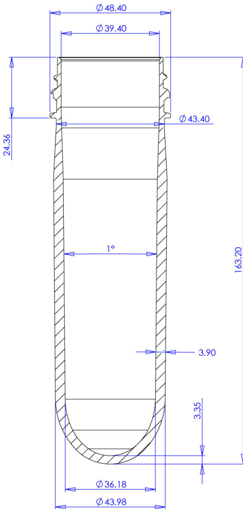
SECTION A-A
